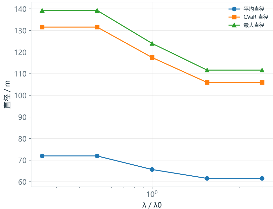
(b) 权重敏感性：定位指标随 \lambda 的变化
